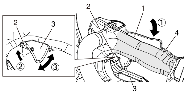
1. Sperrenlösehebel
